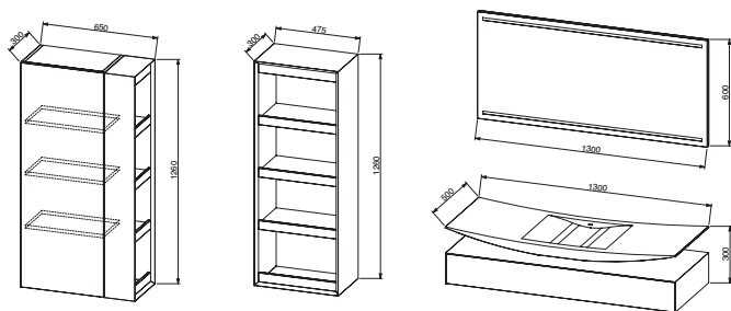
Tehnična slika pohištva Santino 130. Tehnična slika nameštaja Santino 130. Tehnična slika nameštaja Santino 130. Az Santino 130 bútorteknikai képe.
