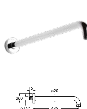
Vintage XL faltámasz készlet. Fali
