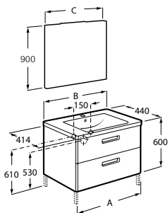
The Gap csomag. Alsószekrény
