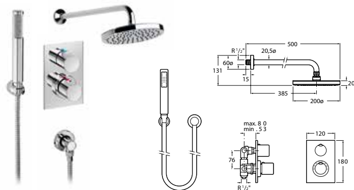
Termosztátos zuhany, beépített, 1/2"
