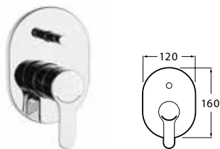
Egykaros kád és zuhany keverőcsap, beépített
