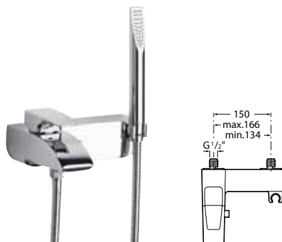
Egykaros fürdőkád és zuhanyzó keverőcsap
