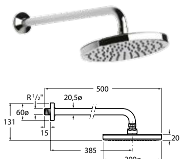
Zuhanykar erős gömbcsuklós fejjel, Ø 200 mm
