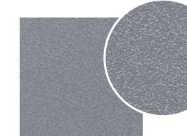
MONO SZARE R płytko gresowa | porcelain tile 200×200×10 mm PÓLMAT | SEMI-MATT QV R10 A *
