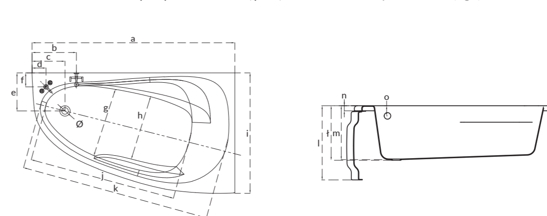
Wanna asymetryczna JOANNA NEW, prawa, lewa JOANNA NEW asymmetric bathtub, right, left
