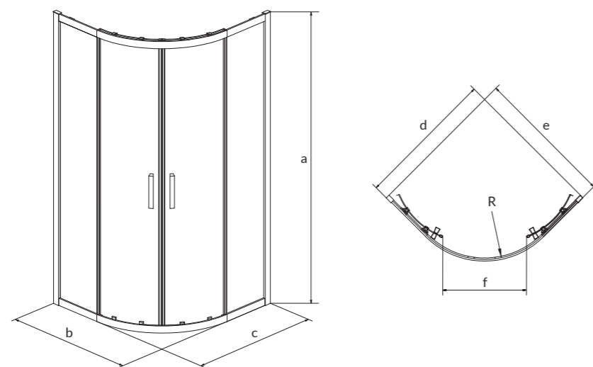
Kabina prysznicowa półokrągła ARTECO ARTECO halfround shower enclosure
