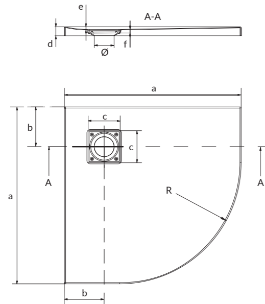
Brodzik półokrągły TAKO SLIM 80, 90 TAKO SLIM 80, 90 halfround shower tray
