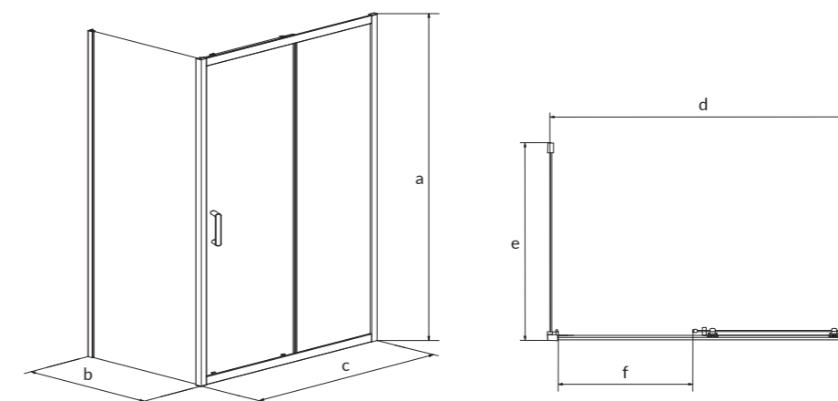
Kabina prysznicowa przesuwna BASIC BASIC sliding shower enclosure
