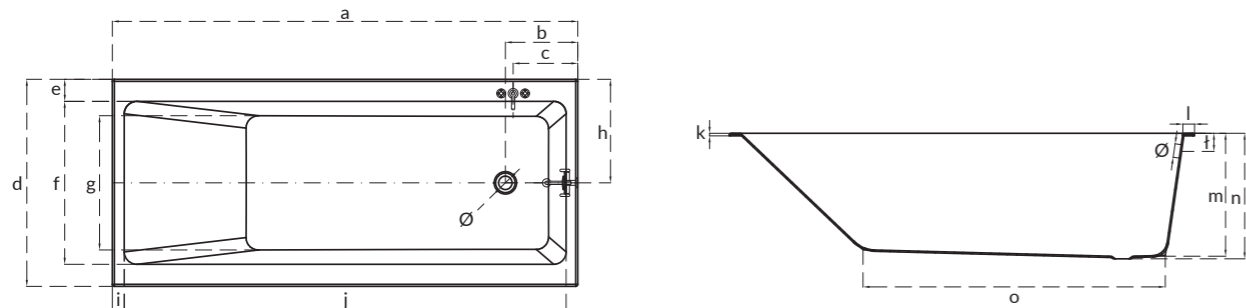
Wanna prostokątna CREA CREA rectangular bathtub
