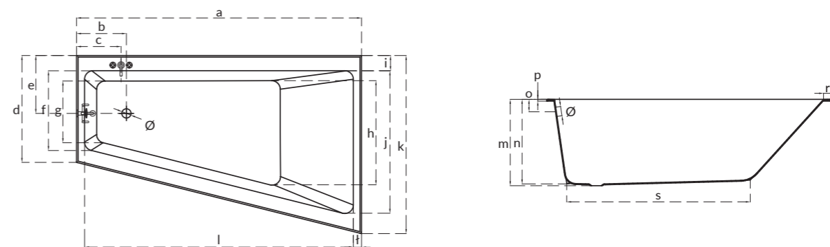
Wanna asymetryczna CREA, prawa, lewa CREA asymmetric bathtub, right, left
