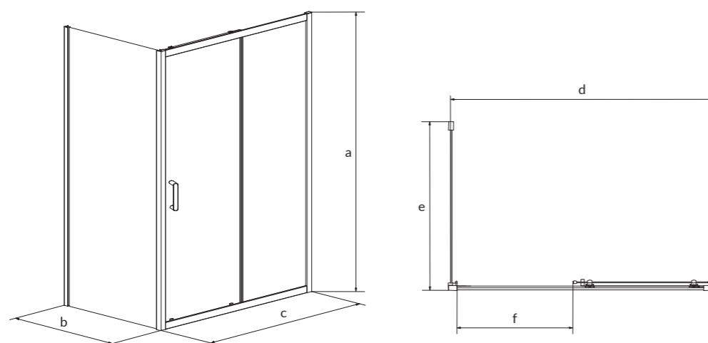
Kabina prysznicowa przesuwna ARTECO ARTECO sliding shower enclosure
