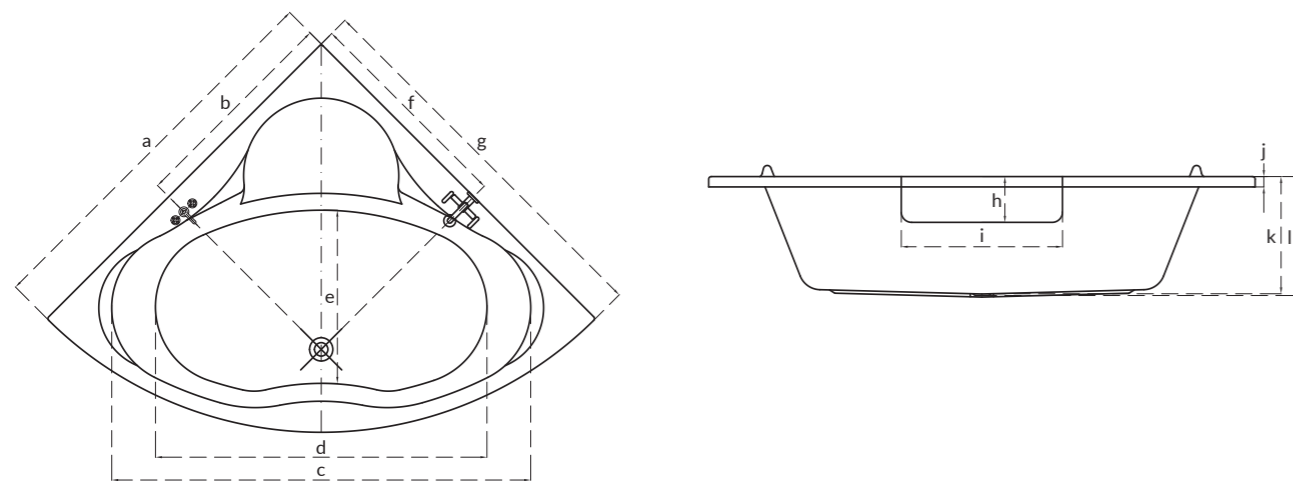
Wanna symetryczna VENUS VENUS symmetric bathtub
