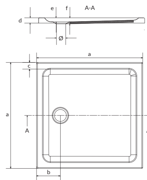
Brodzik kwadratowy TAKO 80, 90 TAKO 80, 90 square shower tray
