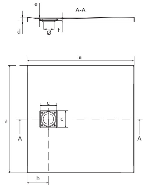
Brodzik kwadratowy TAKO SLIM 80, 90 TAKO SLIM 80, 90 square shower tray
