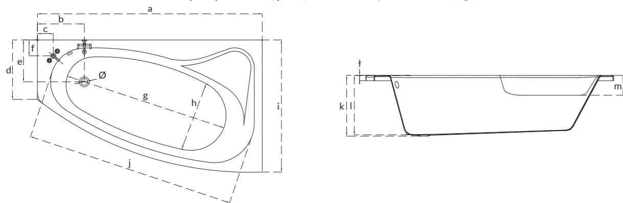
Wanna asymetryczna SICILIA, prawa, lewa SICILIA asymmetric bathtub, right, left
