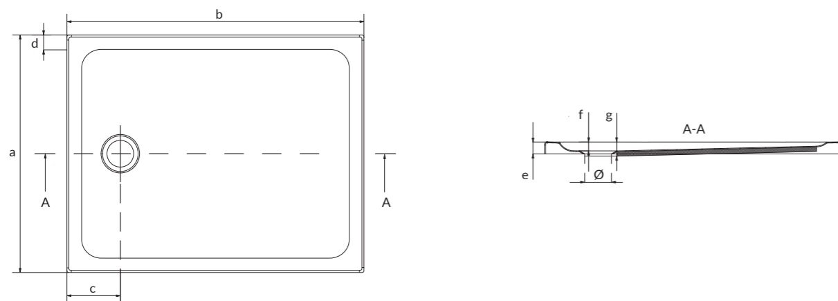
Brodzik prostokątny TAKO 80, 90 TAKO 80, 90 rectangular shower tray
