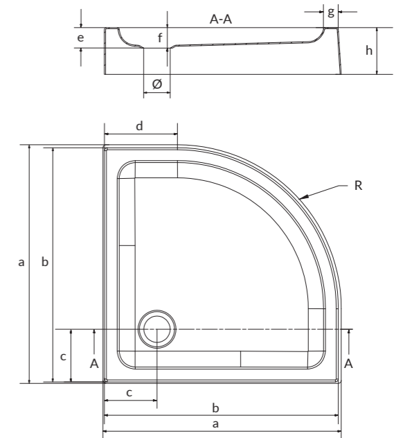
Brodzik półokrągły zintegrowany z panelem TAKO 80, 90 TAKO 80, 90 halfround shower tray built-in-panel
