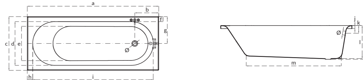
Wanna prostokątna OCTAVIA OCTAVIA rectangular bathtub
