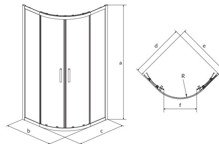
Kabina prysznicowa półokrągła BASIC BASIC halfround shower enclosure
