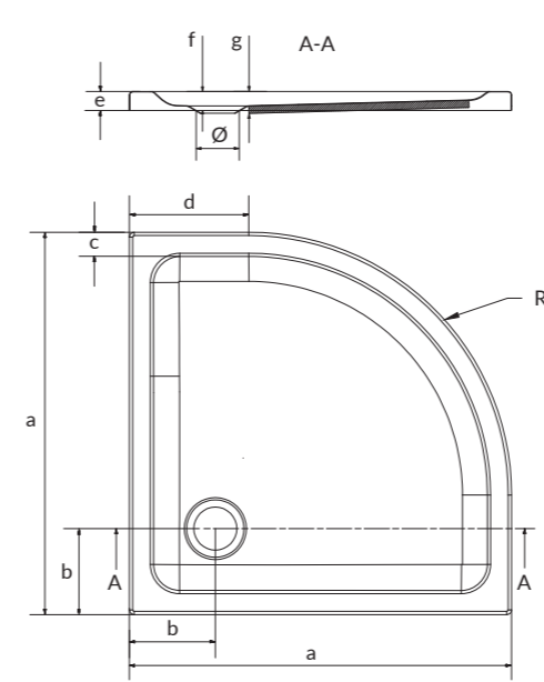
Brodzik półokrągły TAKO 80, 90 TAKO 80, 90 halfround shower tray
