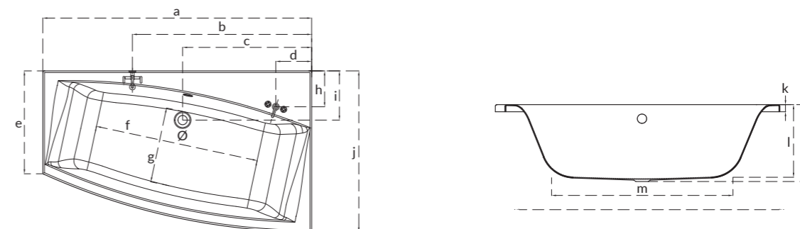
Wanna asymetryczna AIDA, prawa, lewa AIDA asymmetric bathtub, right, left
