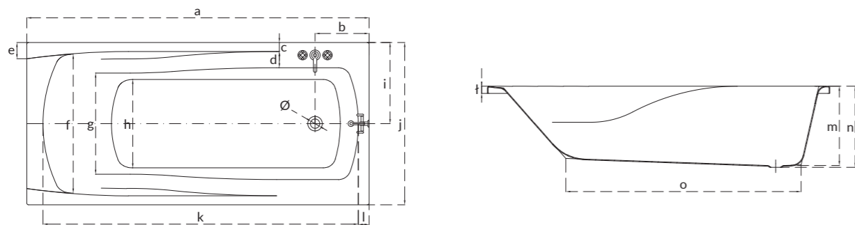
Wanna prostokątna ZEN ZEN rectangular bathtub
