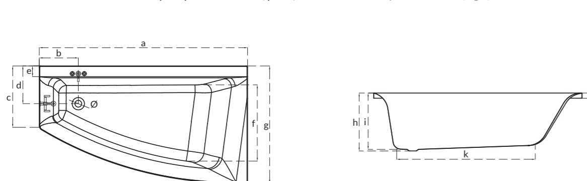
Wanna asymetryczna VIRGO MAX, prawa, lewa VIRGO MAX asymmetric bathtub, right, left
