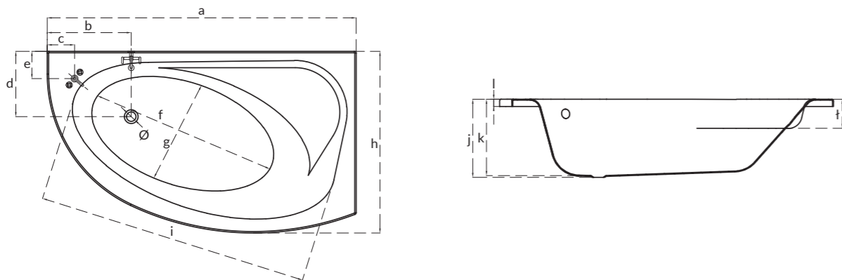
Wanna asymetryczna MEZA, prawa, lewa MEZA asymmetric bathtub, right, left
