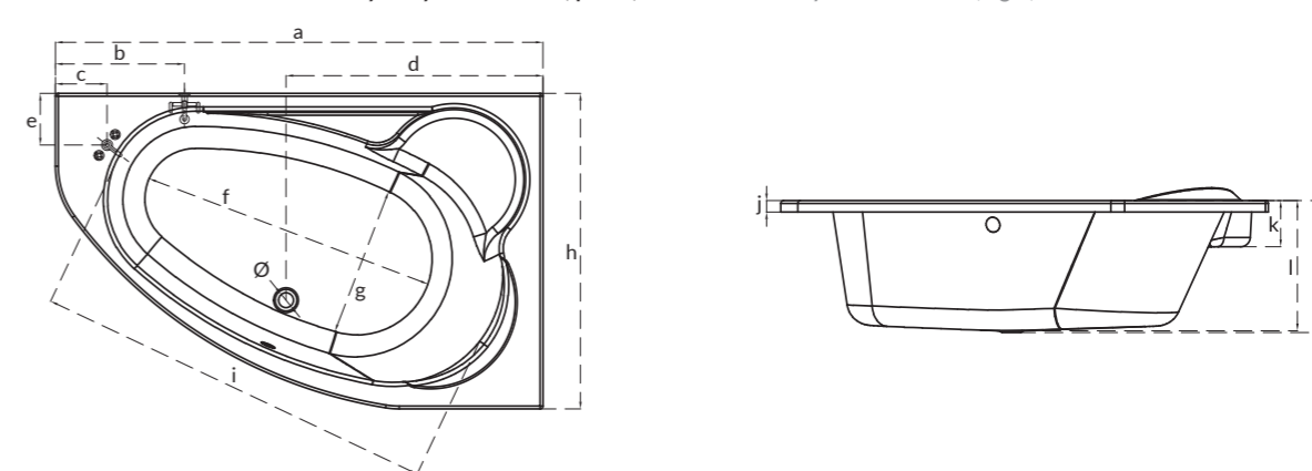
Wanna asymetryczna KALIOPE, prawa, lewa KALIOPE asymmetric bathtub, right, left
