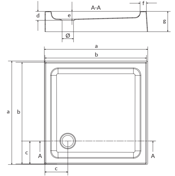
Brodzik kwadratowy zintegrowany z panelem TAKO 80, 90 TAKO 80, 90 square shower tray built-in-panel
