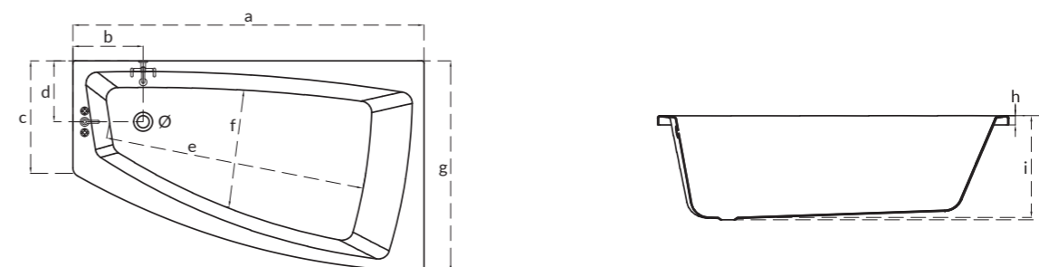
Wanna asymetryczna LORENA, prawa, lewa LORENA asymmetric bathtub, right, left
