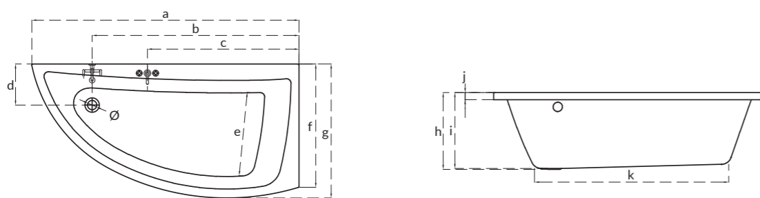
Wanna asymetryczna NANO, prawa, lewa NANO asymmetric bathtub, right, left
